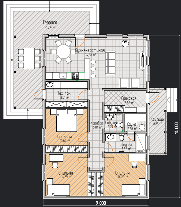
Планировка № 2
